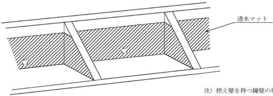
図 3-40(c) 控え壁式擁壁の場合
