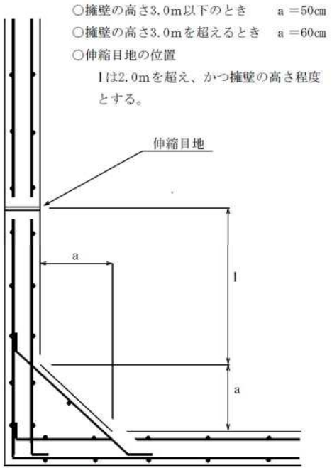
(b) 平面図
