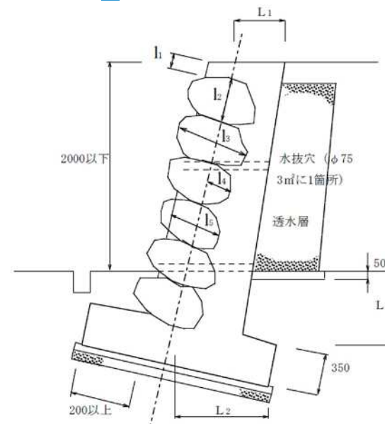
图 3-50
