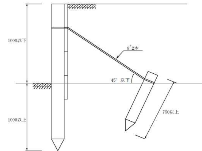
图 3-49
