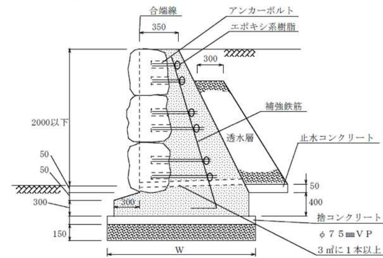
図 3 - 51
